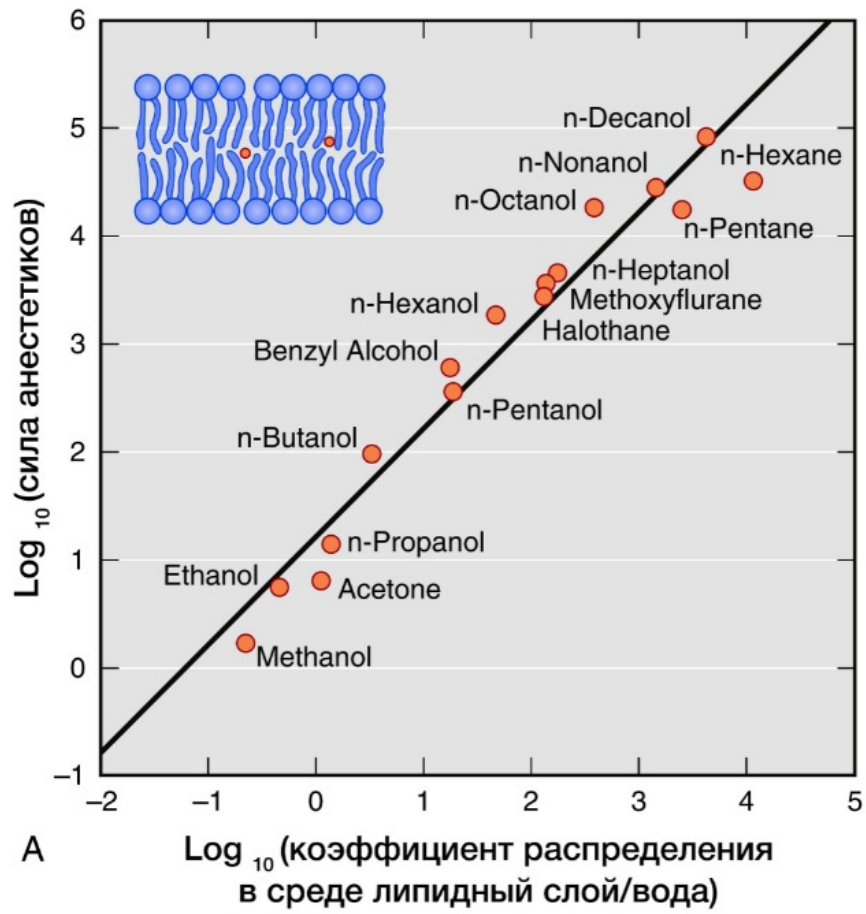
Рисунок 3 | Правило Мейер-Овертона
